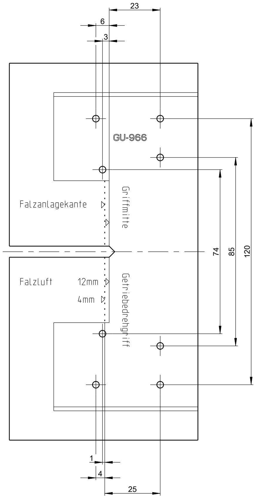
1 x 9-31955-00-0 Bohrschablone für Getriebedrehgriff
